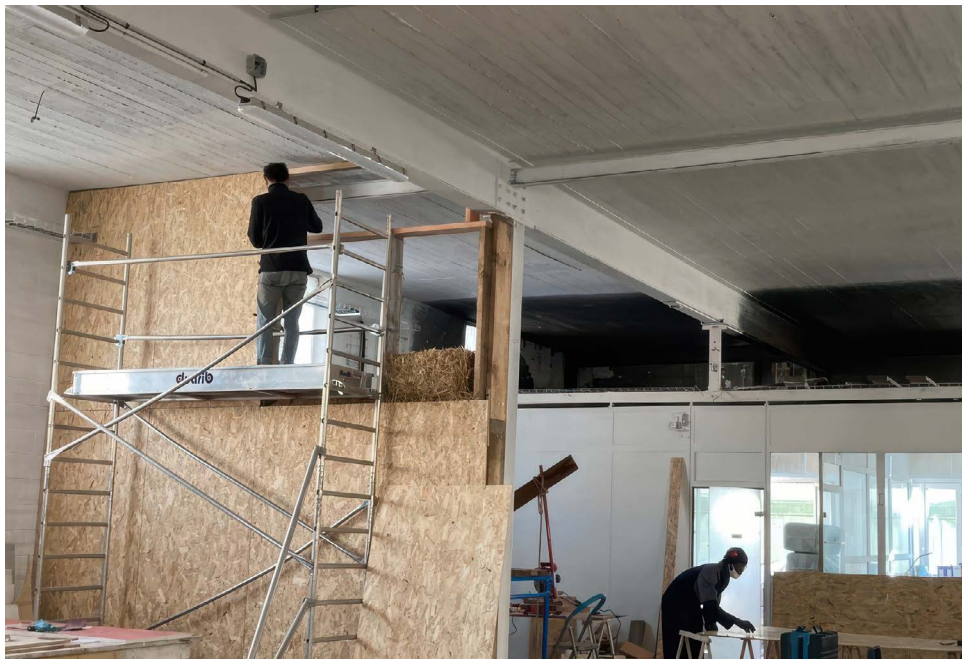
➤ Cloison séparative de l'atelier mutualisé à Romainville (bois récupéré, paille bio, enduit à base de terre récupérée)
